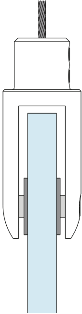
Vue à l'échelle, vitre 5/16po
