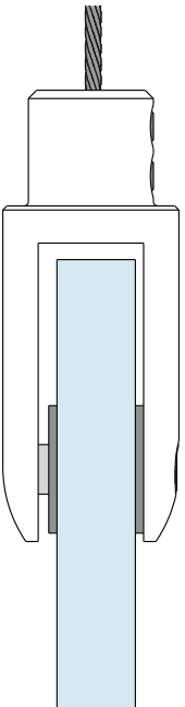
Vue à l'échelle, vitre 3/8po
